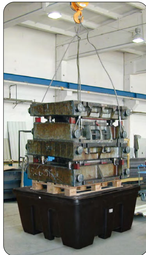
Auffangwanne PE-KT-1S unter einer Prüflast von 8.000 kg
