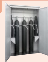
SiZ G30/1200, Artikel-Nr. B80-5017-C, mit seitlichem Einhängeboden, als Zubehör erhältlich
