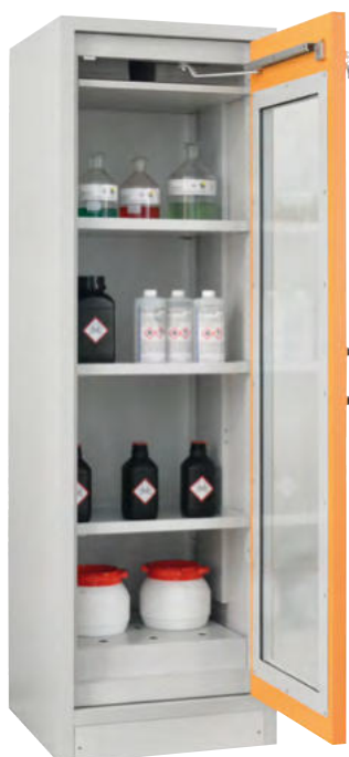
Sis Typ 30 / 600 GL, Artikel-Nr. B80-2655-A, Tür RAL 1007 - narzissengelb, inkl. 3 Einlegeböden, Bodenwanne und Lochblechabdeckung
