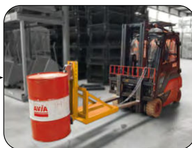
FG 2215/1, RAL 2004 - reinorange, Artikel-Nr. B69-6357-A, L x B x H in mm: 1150 x 600 x 1000, Tragkraft: 400 kg
