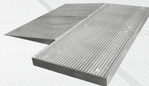
BS 20.10 / 123, Artikel-Nr. P25-1244-B, mit 2 Auffahrrampen AF 10 / 123, Artikel-Nr. P25-1261-B und Rampen- verbinder RV 123, Artikel-Nr. P25-1256-B
