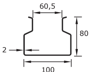
Typ KSL 20 max. Feldlast 12 t*
