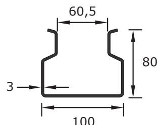
Typ KSL 30 max. Feldlast 17 t*
