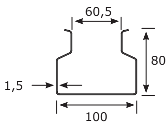
Typ KSL 15 max. Feldlast 9 t*
